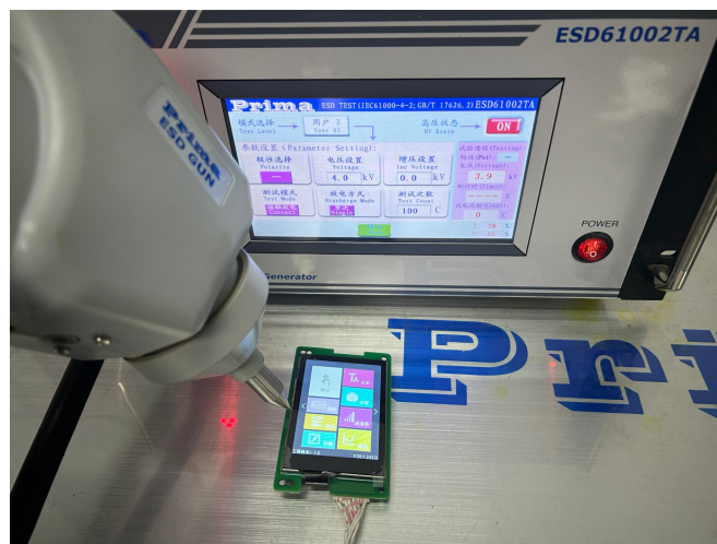
图 4-2 ESD 测试图
