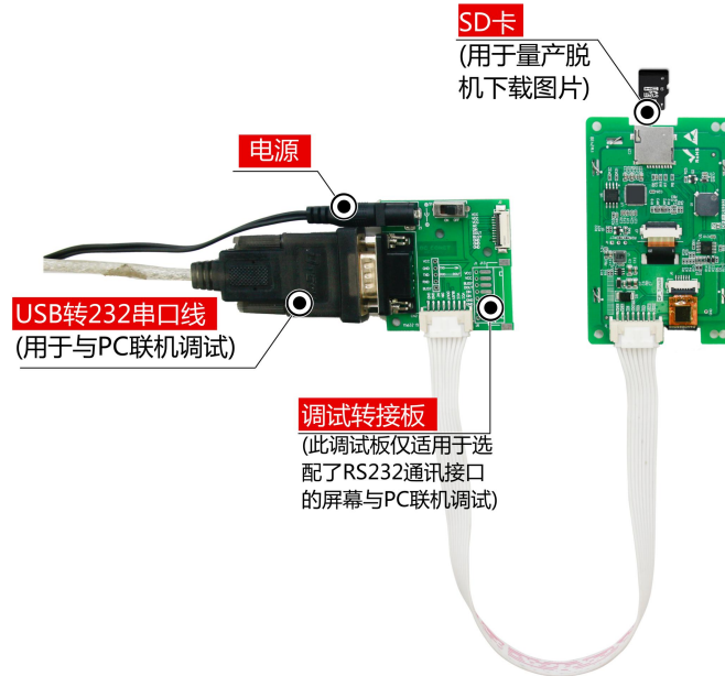
图 1-4 调试工具图
