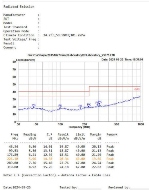
图 4-5 RE 测试水平方向
